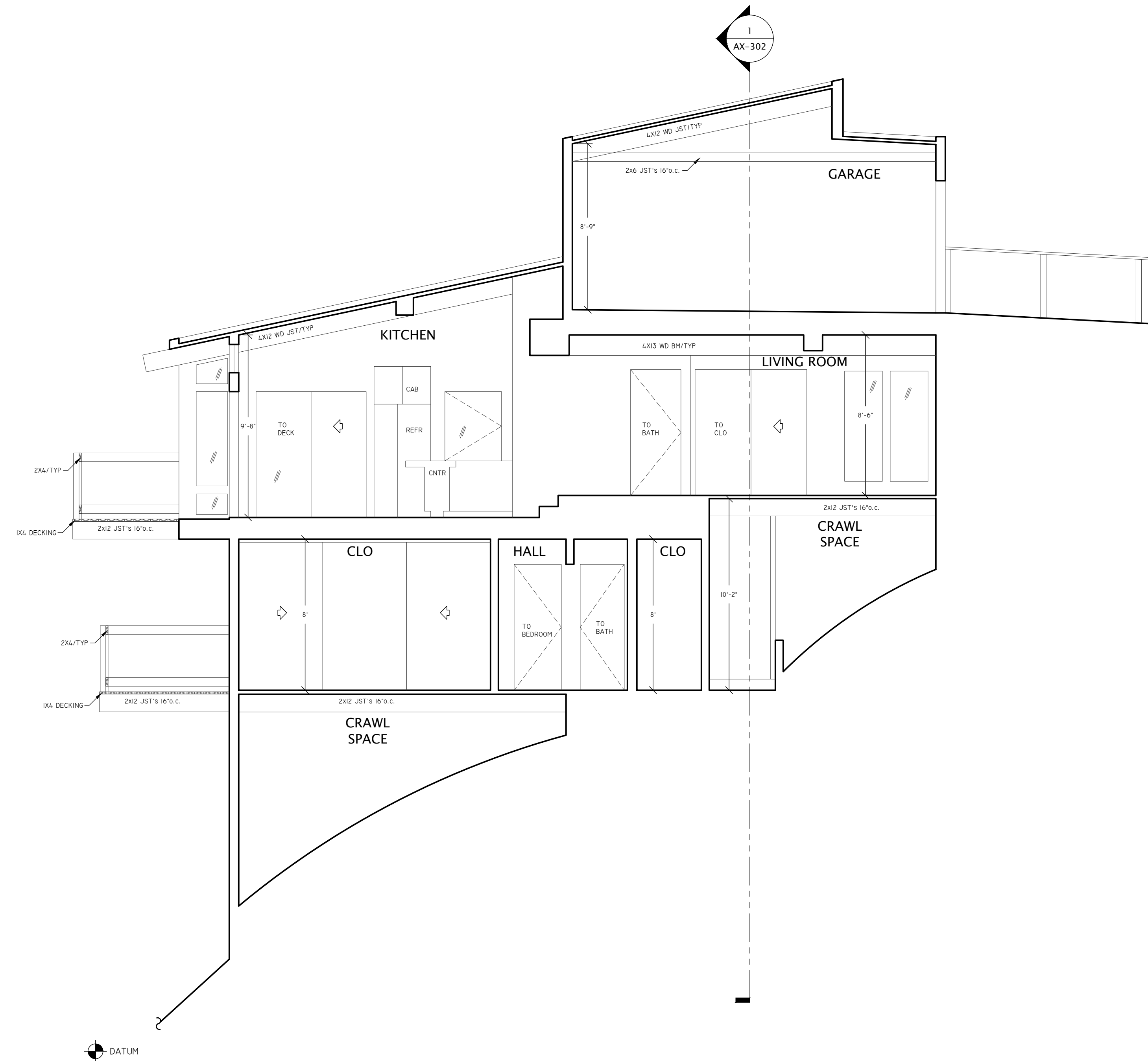
1 EXISTING LONGITUDINAL SECTION
